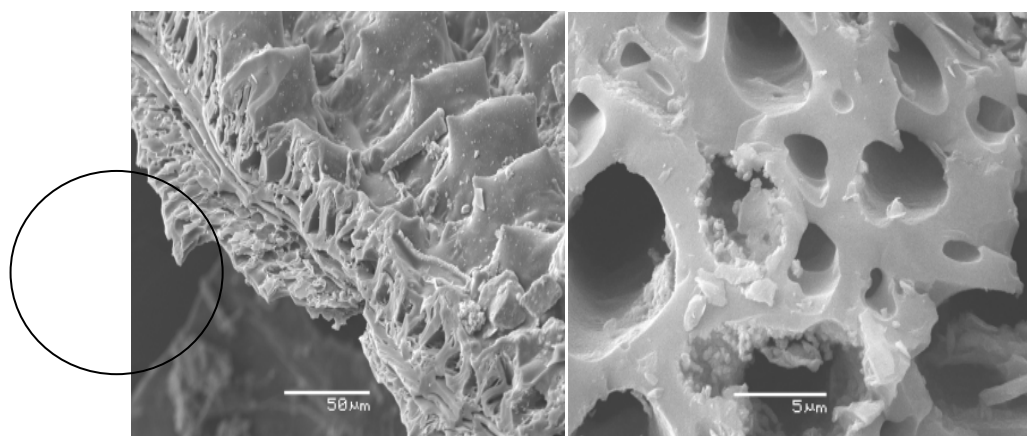
Рисунок 1 – Снимки образцов КРШ полученных методом СЭМ
