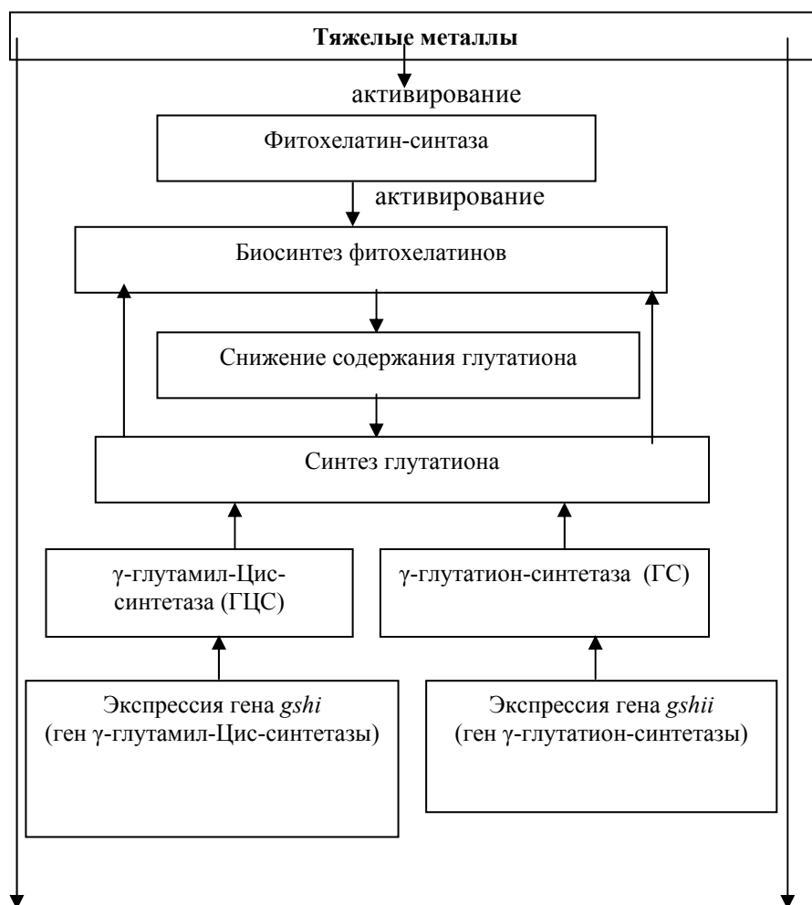
Рисунок 1 – Схема регуляции синтеза фитохелатинов в растениях
